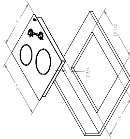
Modelos: ARKIC2, ANHANCIC2 & GUA-CIER2
