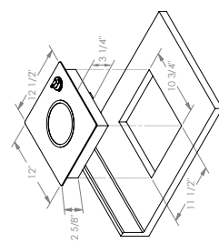
Modelos: MED1, CAR1, ALP1, COR1
